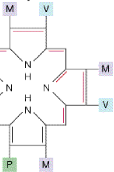
Protoporphyrin IX
