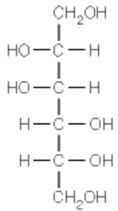
D-Mannitol
