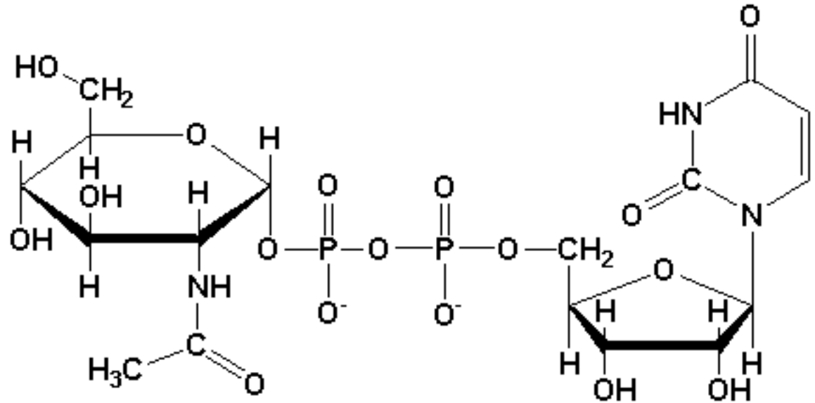
UDP-N-acetylgalactosamine
