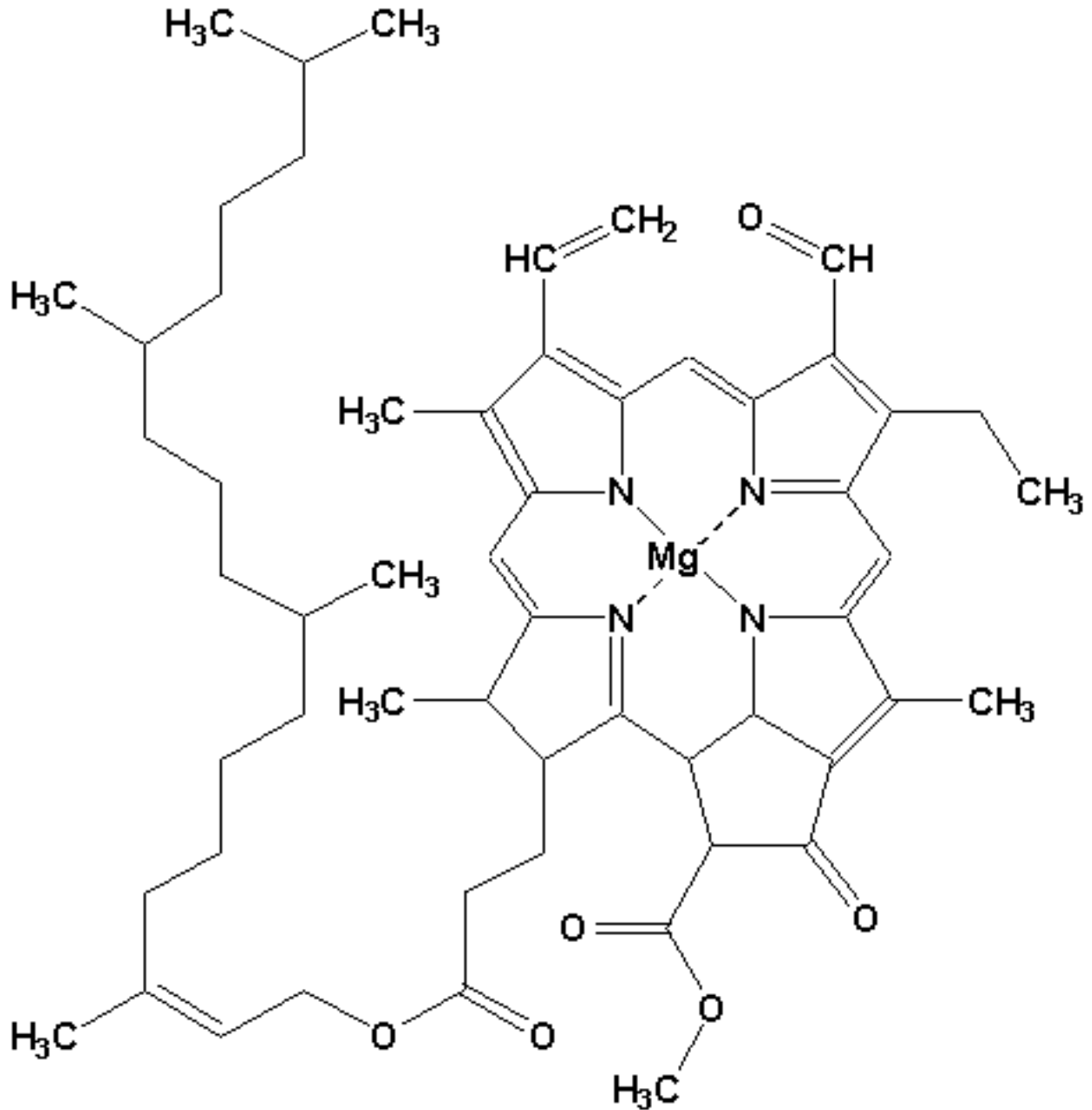
Chlorophyll B
