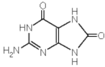
8-Oxoguanine
