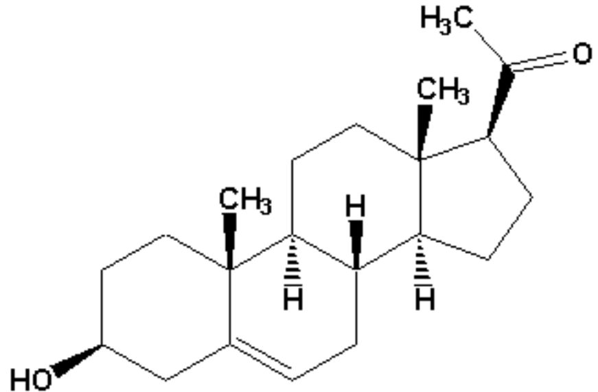
Pregnenolone
