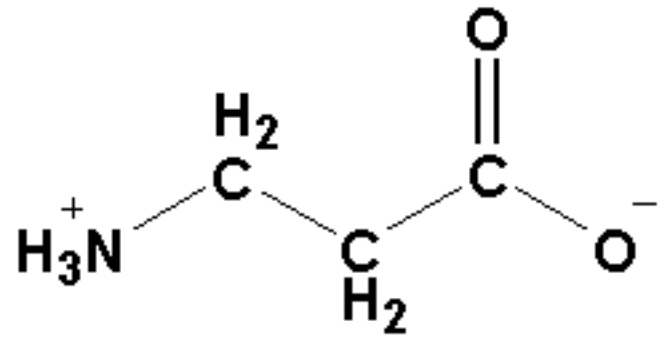
Beta-alanine
