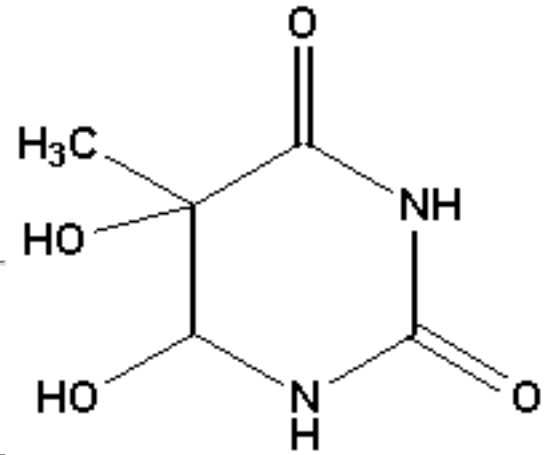
Thymine glycol
