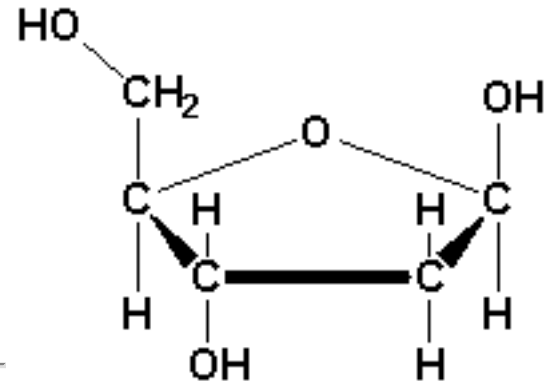
Deoxyribose
