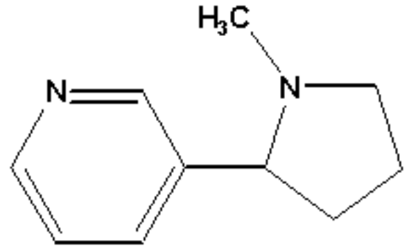
Nicotine
