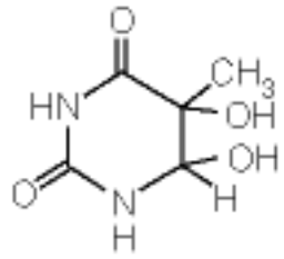
Thymine glycol
