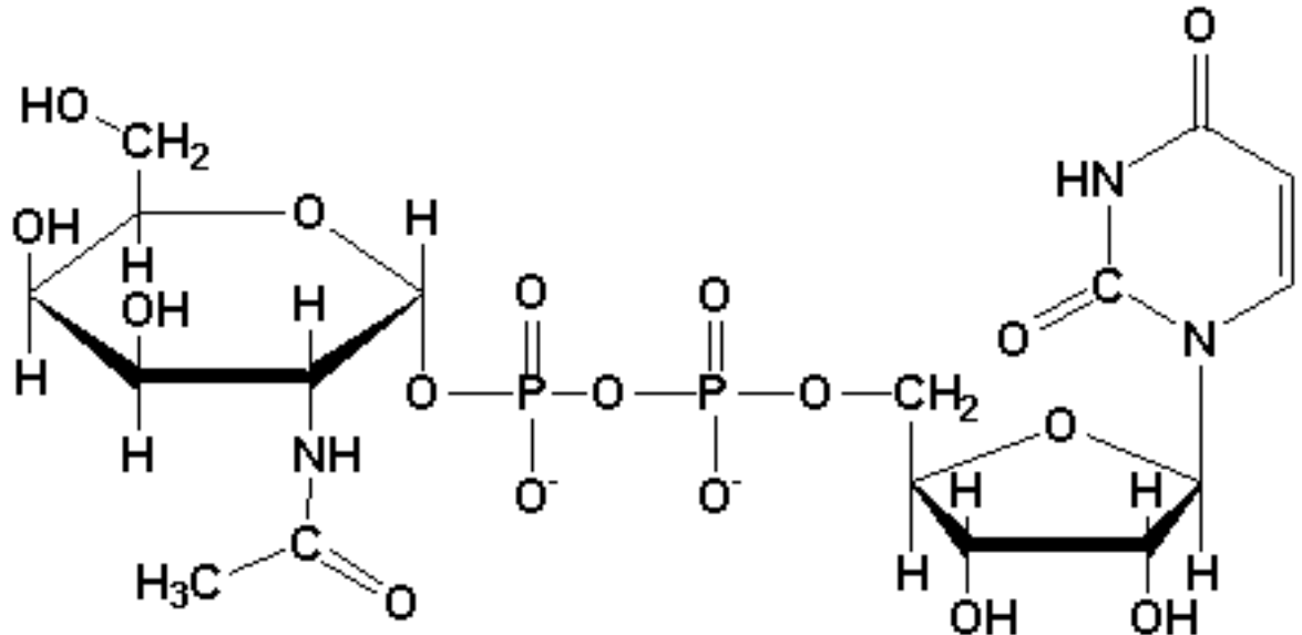
UDP-N-acetylgalactosamine
