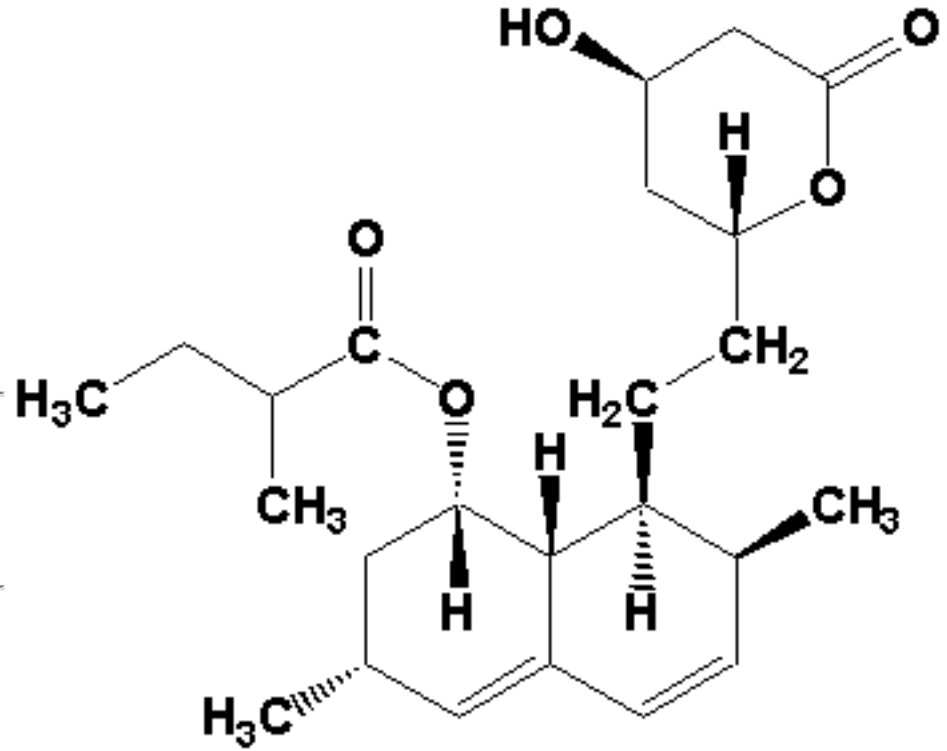
Lovastatin
