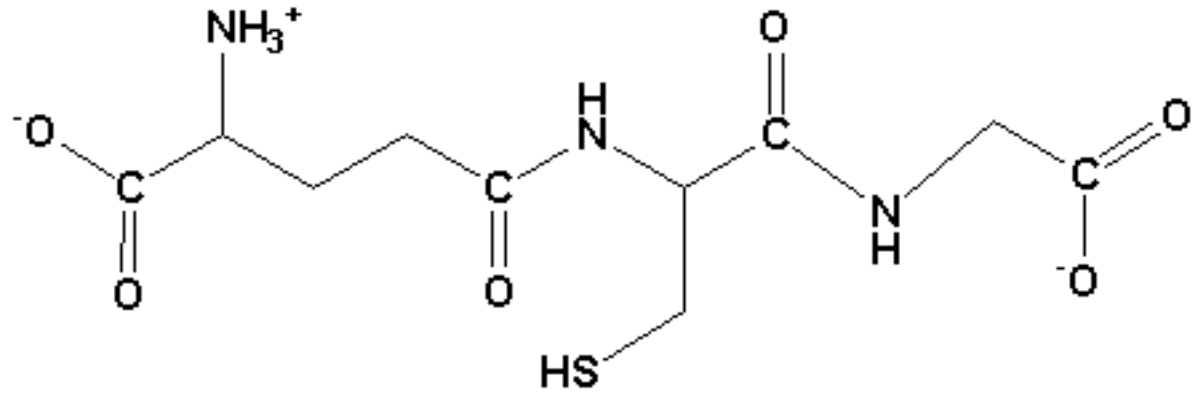
Glutathione
