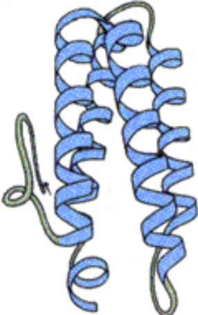
Myohemerythrin
