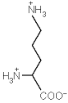
Ornithine
