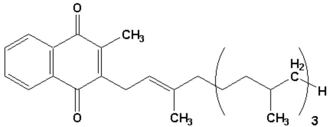
Phylloquinone A1
