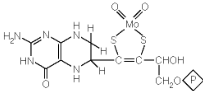
Molybdopterin
