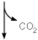
Ornithine
