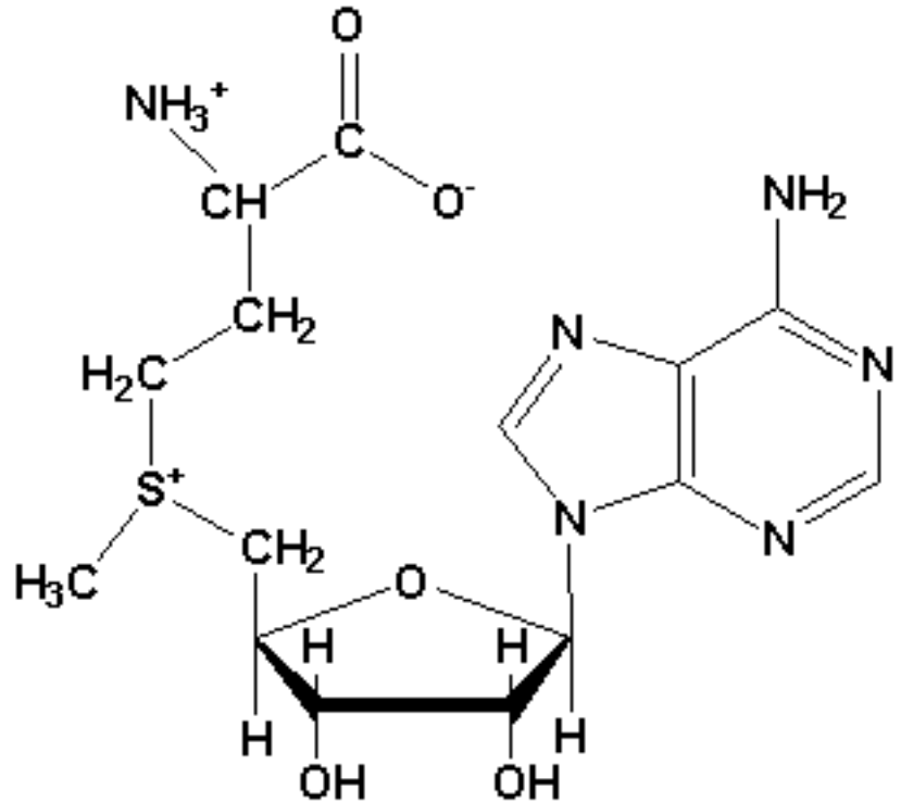
S-Adenosylmethionine (S-AdoMet)
