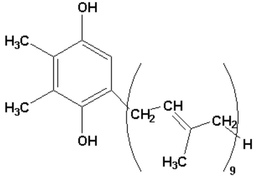
Plastoquinone QH 2
