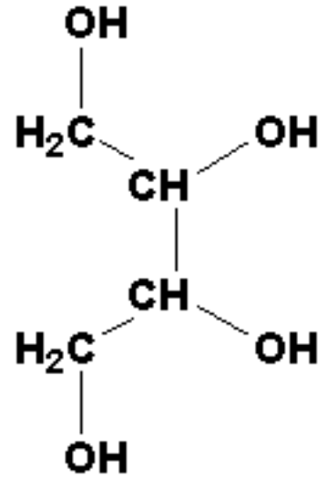
Erythritol
