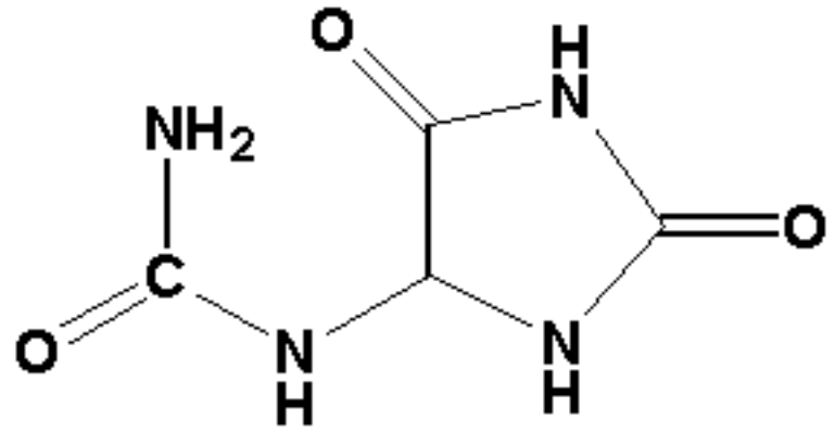
Allantoin
