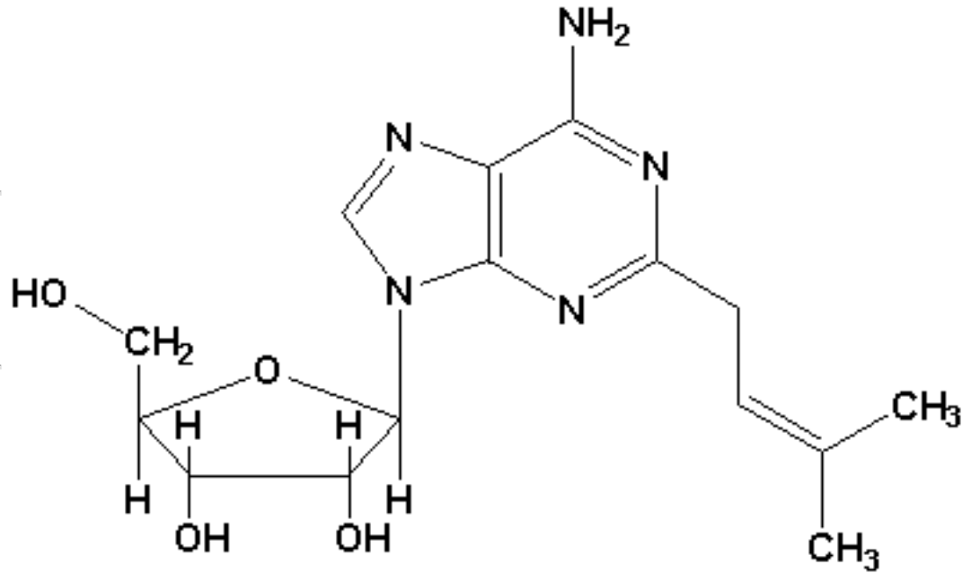
2-Isopentenyladenosine
