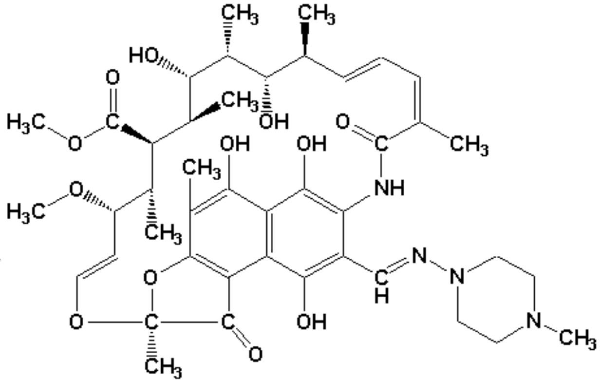
Rifampicin
