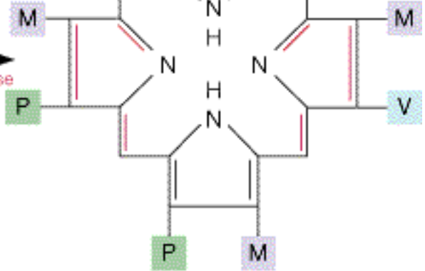
Protoporphyrin IX
