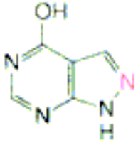
Allopurinol
