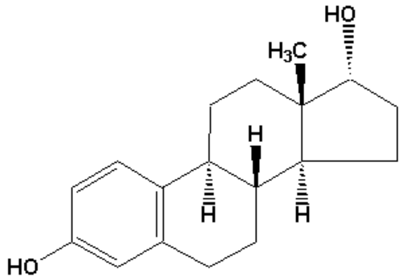
Estradiol(alpha)
