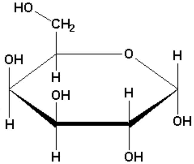
Galactose
