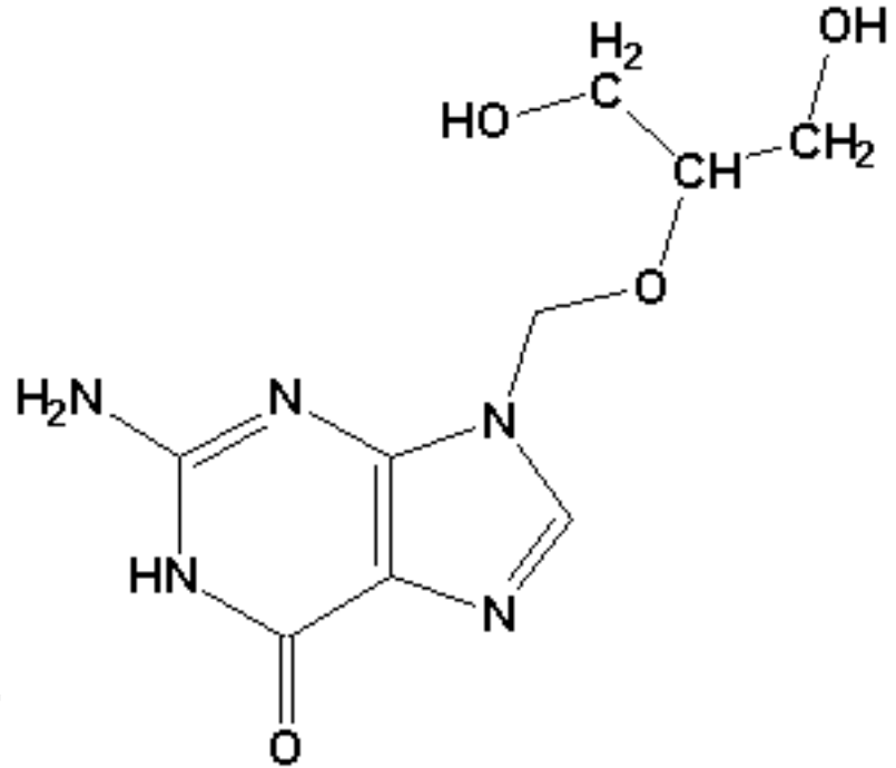
Ganciclovir
