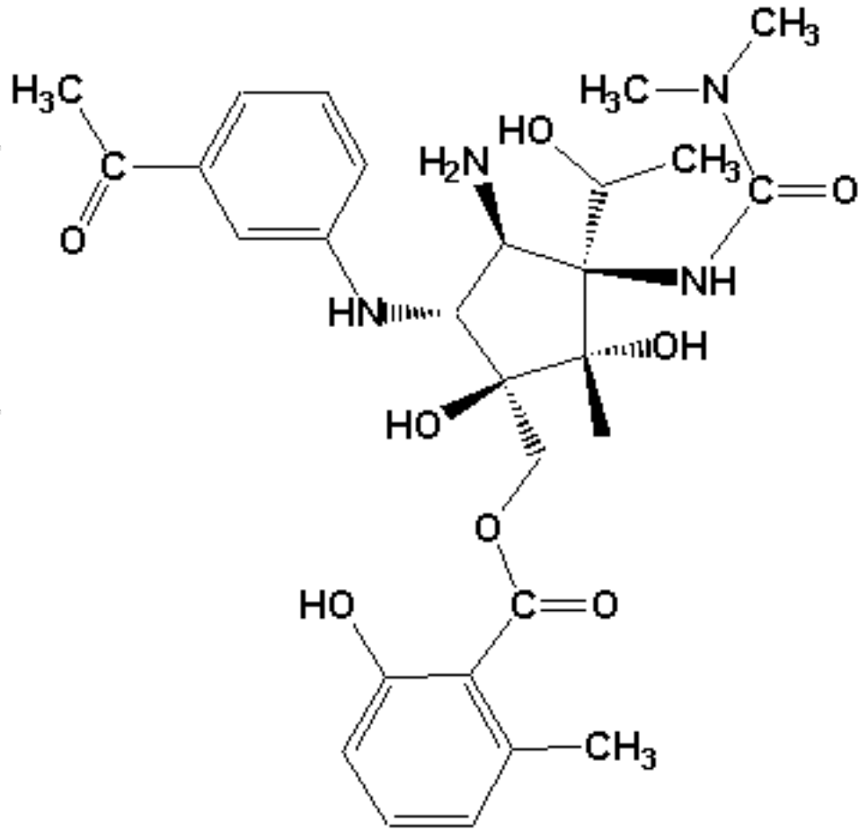
Pactamycin
